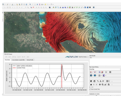
Storm Tide Result Visualisation
